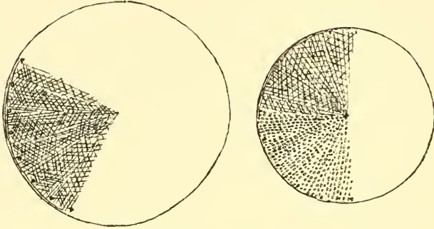
Fig. 6. Coscinodiscus Joergensenii n. nom. 500 t. m.
