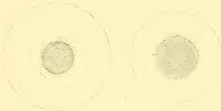
Fig 1. Hyalodiscus laevis Ehrbg. 250 t. m.
