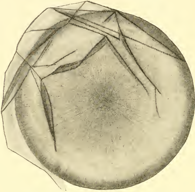
Fig. 4. Coscinodiscus subbulliens Jørg. 250 t. m.
